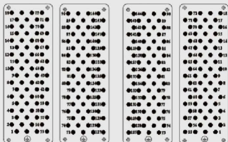
接插针排序
